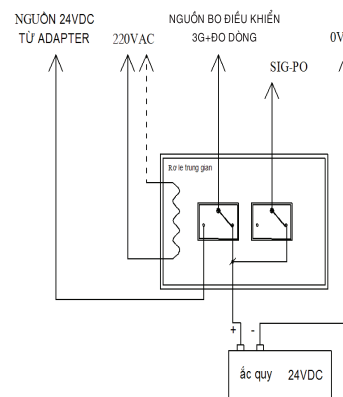
Hình 5: sơ đồ nguồn cấp cho mạch điều khiển bổ sung
