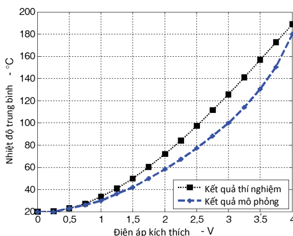
Hình 10: nhiệt độ trung bình vi kẹp theo điện áp kích thích trên mỗi thanh chấp hành
