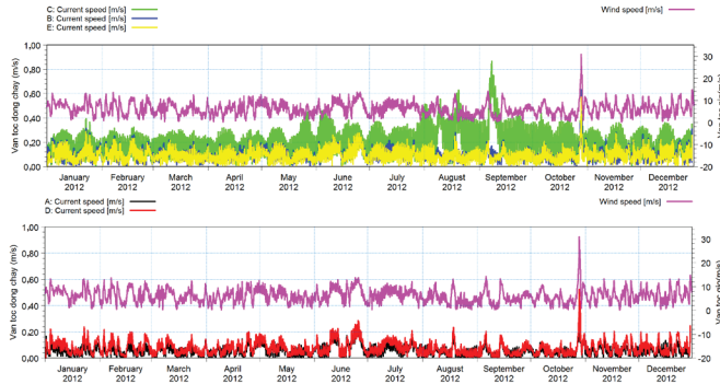
Hình 10: vận tốc dòng chảy tại các điểm trong năm 2012
