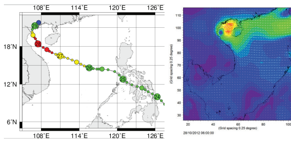
Hình 14: đường đi và trường gió của cơn bão Sơn Tinh (bão số 8 năm 2012) Nguồn: Tổ chức khí tượng Nhật Bản và ECMWF
