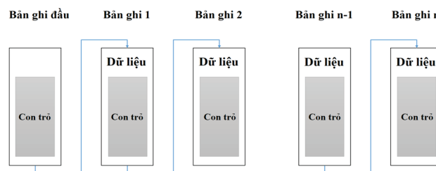
Hình 1. Kiến trúc của Blockchain [5].
