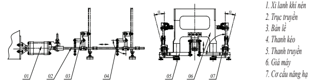
Hình 3: sơ đồ cấu tạo cơ cấu xoay giá kẹp
