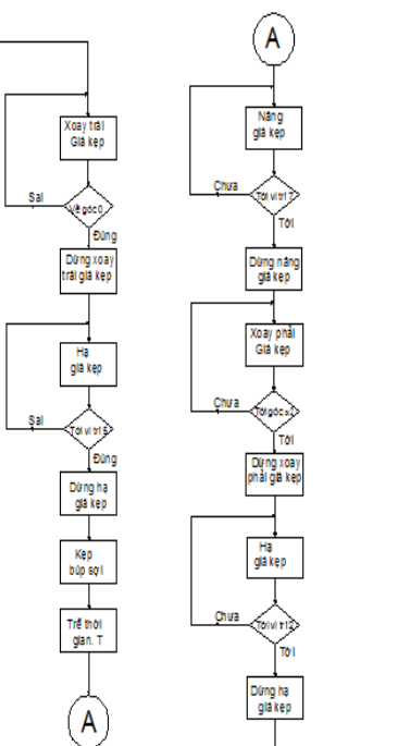
Hình 7: lưu đồ điều khiển đưa ống sợi xuống băng truyền
