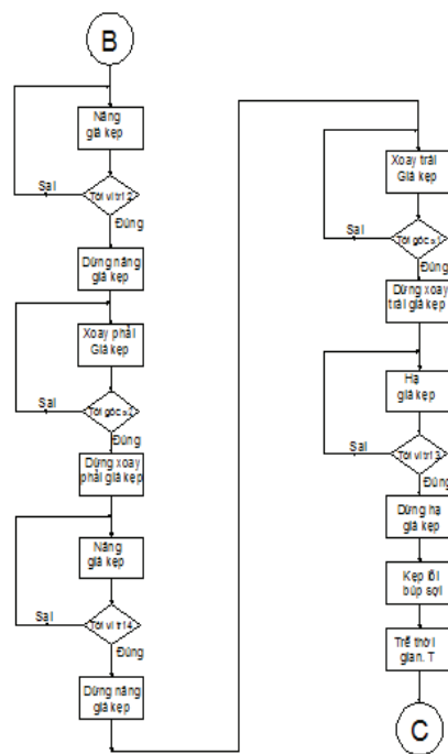
Hình 8: lưu đồ điều khiển đưa giá kẹp lên giá trung gian
