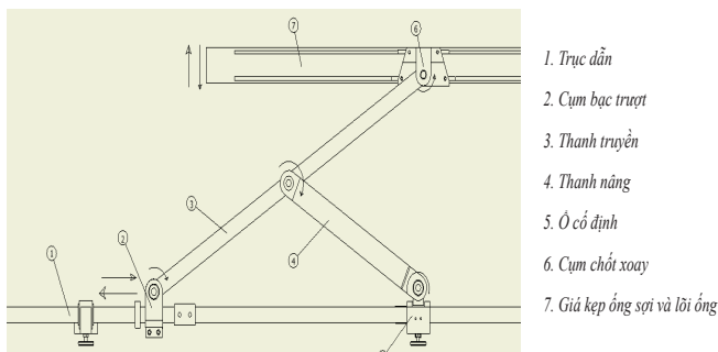
Hình 2: sơ đồ cấu tạo cơ cấu nâng - hạ giá kẹp
