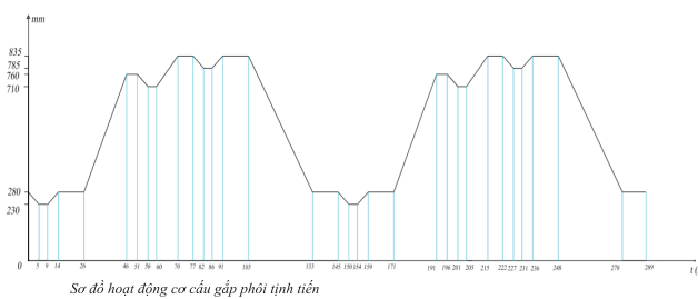
Hình 11: đồ thị chu trình đồ sợi
