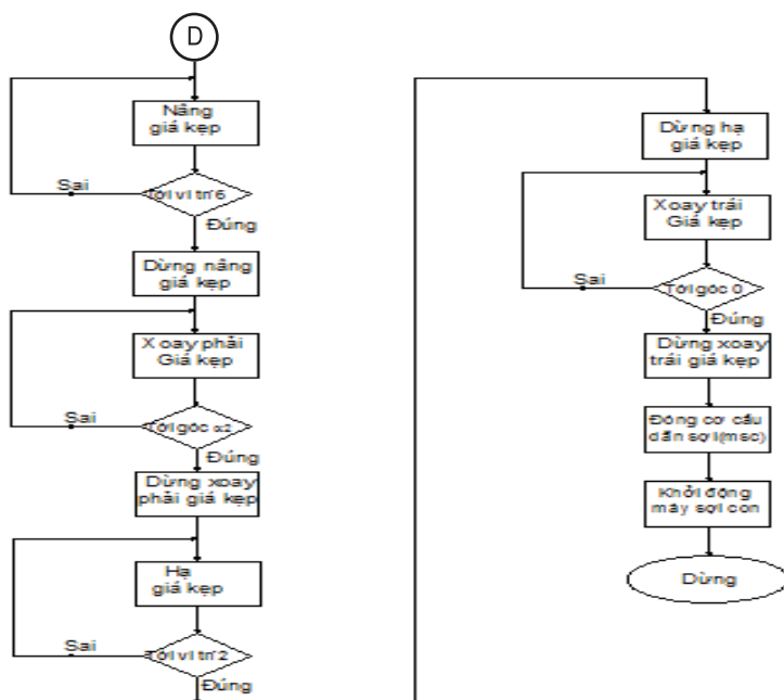
Hình 10: lưu đồ điều khiển đưa giá kẹp về vị trí chờ
