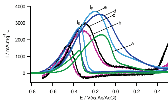
Hình 3. Đường quét dòng thế tuần hoàn (CV) của các xúc tác: a- Pt_{20,5}/rGO , b- Pt_{2,5}Co_{14}/rGO , c- Pt_{2,4}Ni_{11,1}/rGO , d- Pt_{22,1}Al_{1,7}Si_{3,1}/rGO và e- Pt_{11,5}Al_{12,7}/rGO (NaOH 0,5M, etanol 1M, 50 mV/s).
