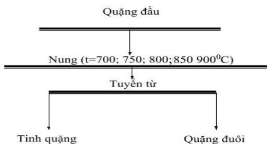
Hình 1: sơ đồ nung - tuyển từ quặng đuôi mẫu CNBL-I cấp hạt M < 2 ở các cấp nhiệt độ khác nhau
