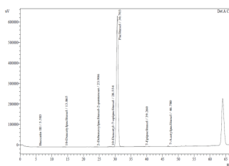
Hình 6: sắc ký đồ mẫu chuẩn PTX và tạp chuẩn B
