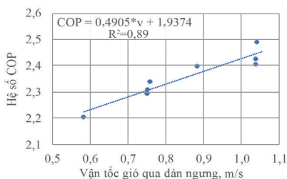
Hình 4. Quan hệ giữa vận tốc gió vào dàn ngưng và hiệu quả biến đổi năng lượng của chu trình.
