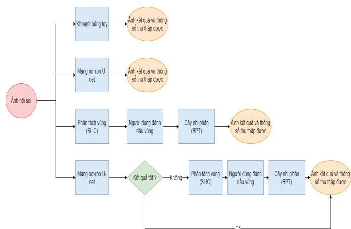
Hình 1. Sơ đồ khối cách vận hành của phần mềm so sánh 4 chế độ khoan đường Z.
